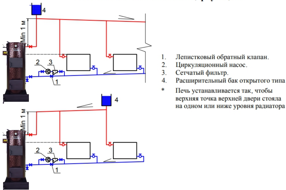
Рис.7 Система с естественной циркуляцией
