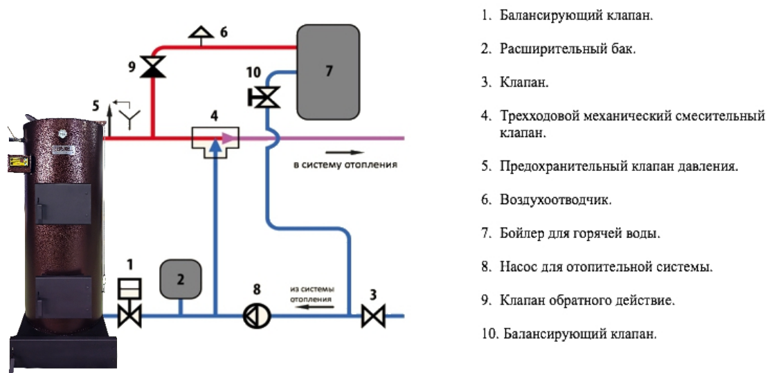
Рис.4 Рекомендуемая схема (бойлер параллельно)
