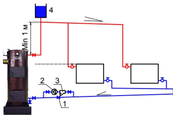
Рис. 6 Система с естественной циркуляцией (попутная)
